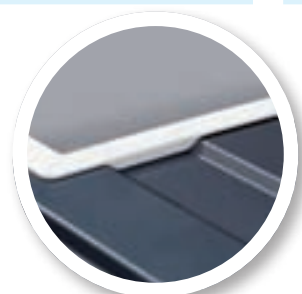
Inbouwframe voor airconditioning of dakraam op een dak van trapeziumplaat
