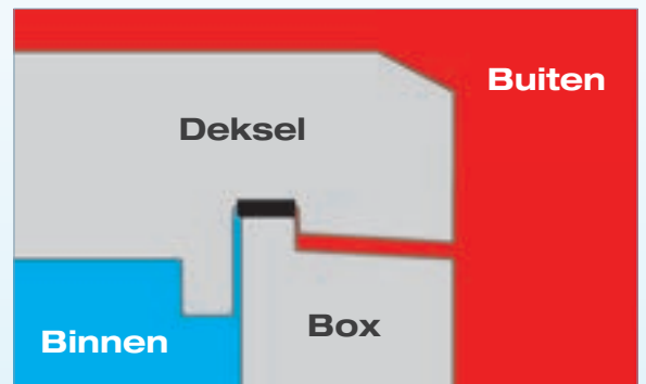
De labyrintafdichting verhindert het binnendringen van warmte in de koelbox.
